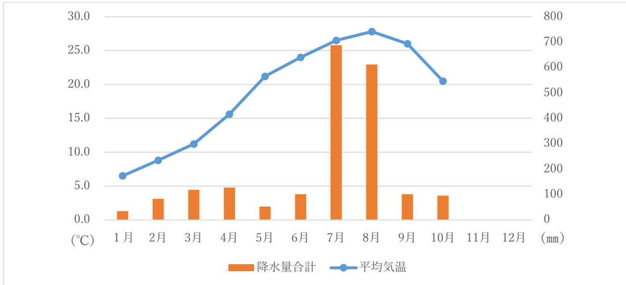
第 8 図 令和元年の気候データ（気象庁久留米観測地点）
